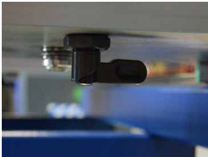
FERMO DI PIANO ROTANTE
